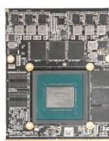
NVIDIA RTX 3500 ADA MXM 3.1 Type B
